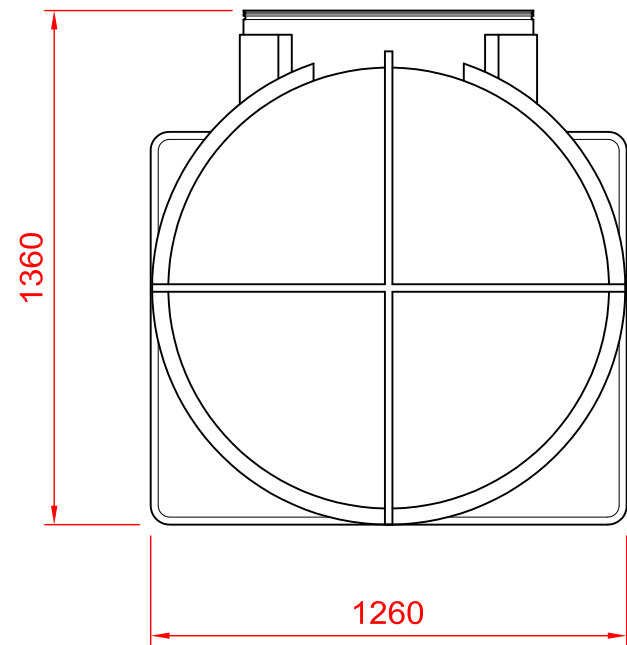
END ELEVATION
